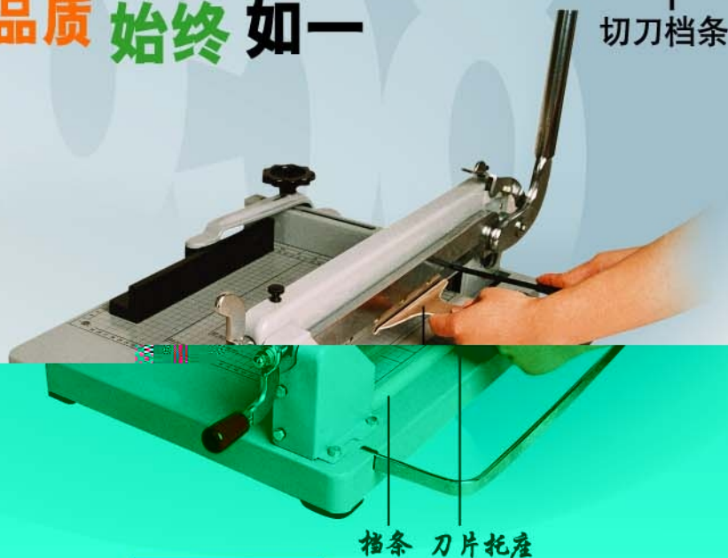
部件标图 2
